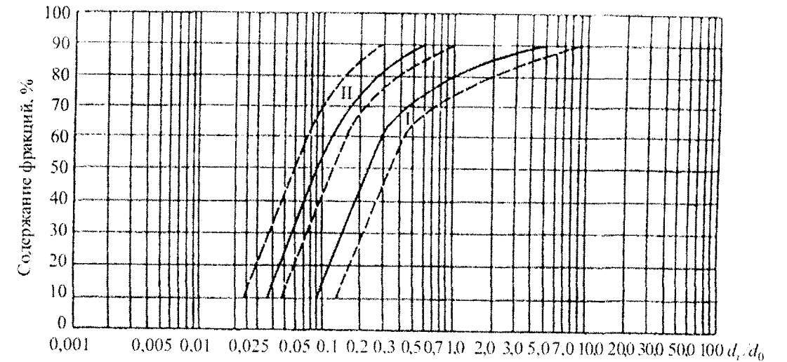
Рисунок E.2 – График зависимости \alpha = f\left(\frac{d_i}{d_0}\right) для неоднородных плотин из мелкого песчано-гравийного грунта с центральной песчаной зоной
