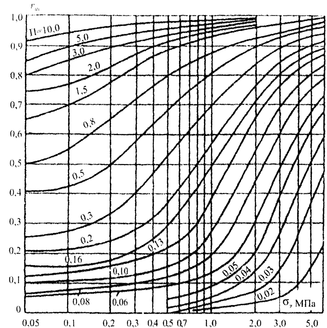
Рисунок А.1 – Номограмма для определения порового давления r_{uc}
