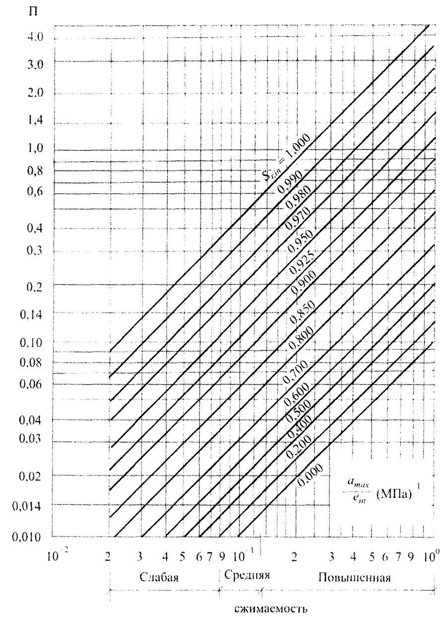
Рисунок А.2 – Номограмма для определения параметра П
