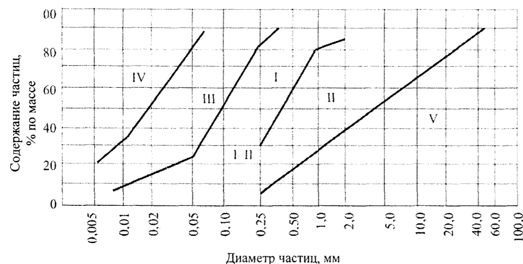
Рисунок 6 – Группы грунтов, используемых для намыва плотин
