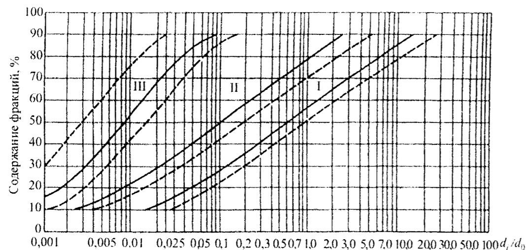
Рисунок E.5 – График зависимости \alpha = f\left(\frac{d_i}{d_0}\right) для гравийных плотин с ядром высотой > 30 м
