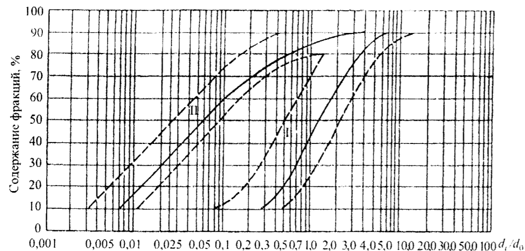
Рисунок E.4 – График зависимости \alpha = f\left(\frac{d_i}{d_0}\right) для гравийных плотин с ядром высотой < 30 м
