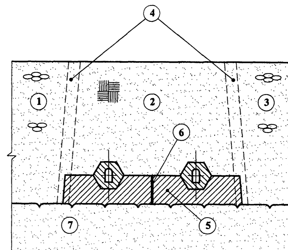
1 – верхняя призма плотины; 2 – ядро плотины; 3 – нижняя призма плотины; 4 – переходные слои; 5 – бетонная пробка с галереями; 6 – температурно-деформационные швы; 7 – скальное основание
