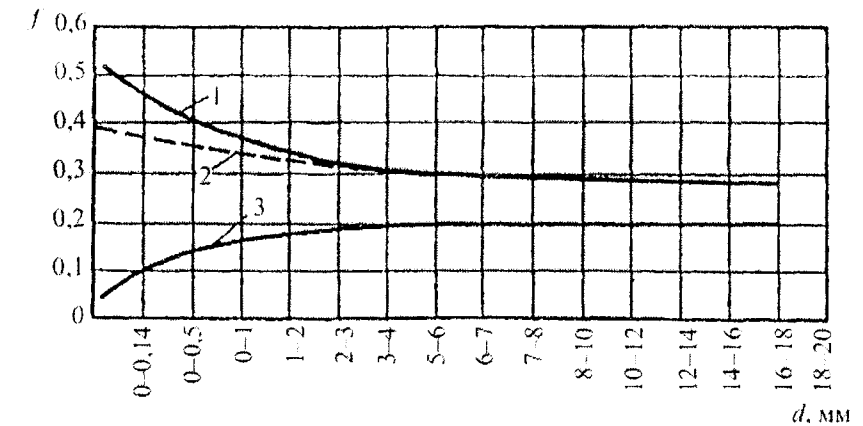
Рисунок Ж.3 – Зависимость коэффициента трения грунтов по стальной диафрагме от их крупности и влажности
