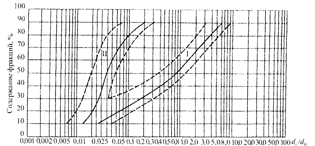
Рисунок E.2 – График зависимости \alpha = f\left(\frac{d_i}{d_0}\right) для неоднородных плотин из мелкого песчано-гравийного грунта с центральной песчаной зоной
